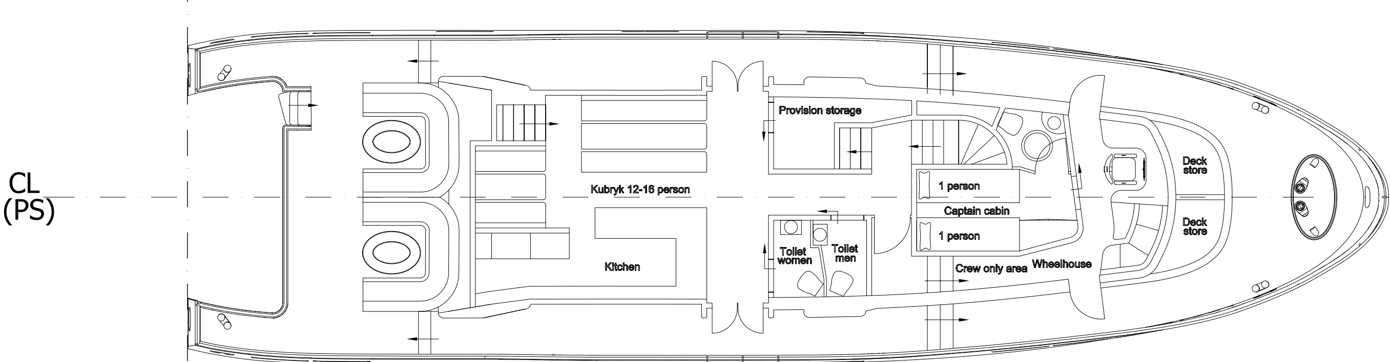
View on Main Deck (Widok na Pokład Główny)
