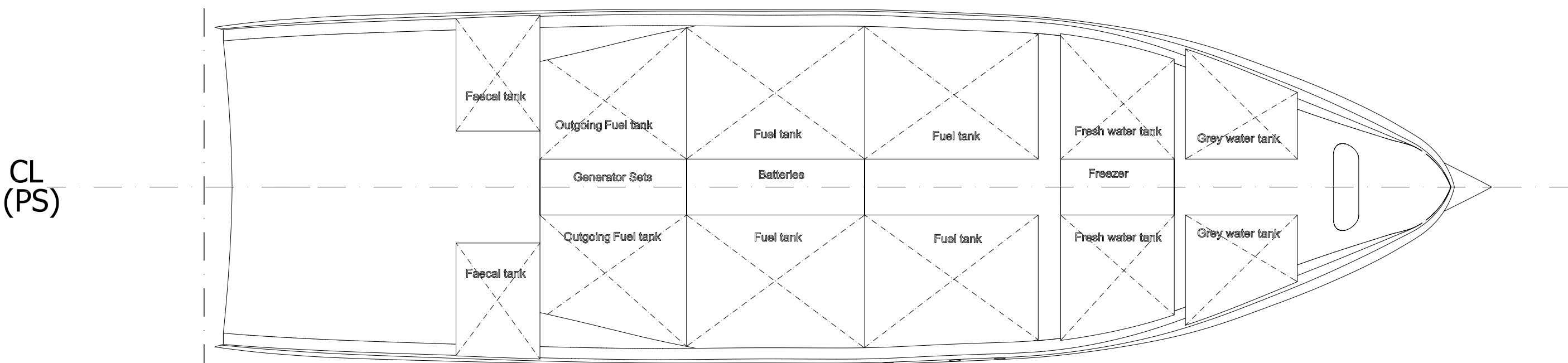
Tank plan (Plan zbiorników)
