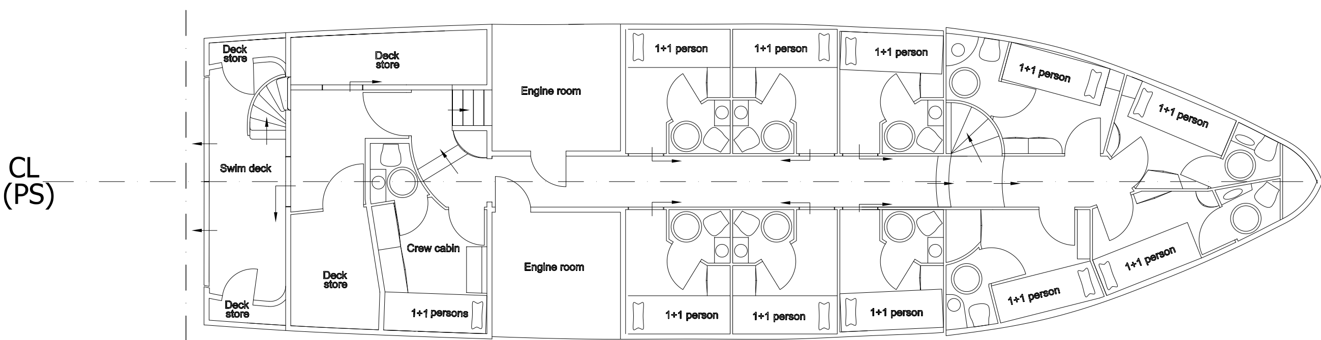
View below Main Deck (Widok pod Pokładem Głównym)
