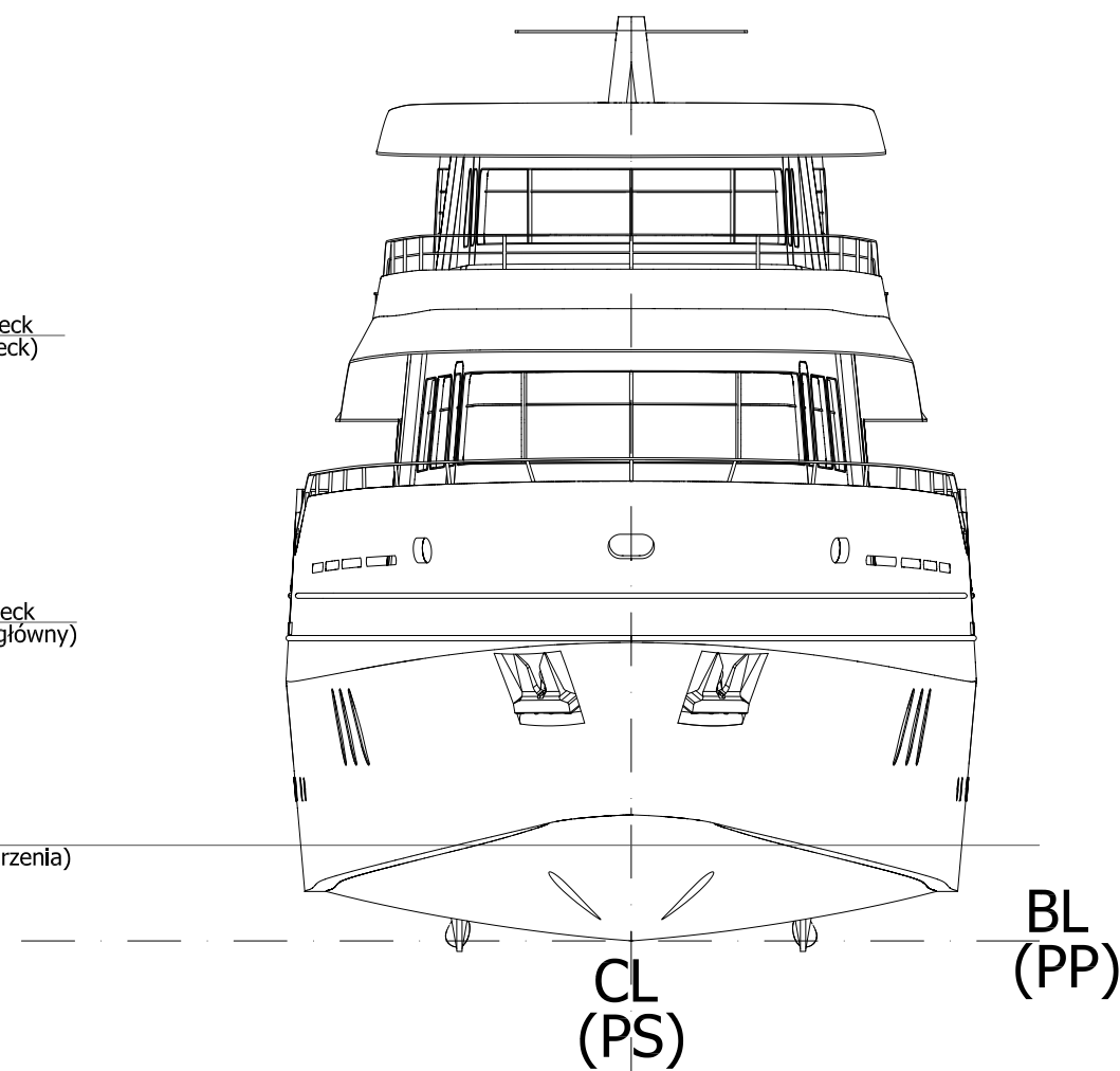
Bow view (Widok od dziobu)
